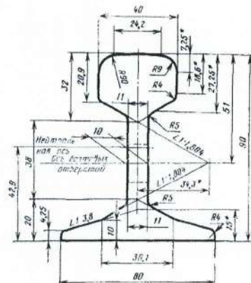
Рис. 2 Рельс Р18
